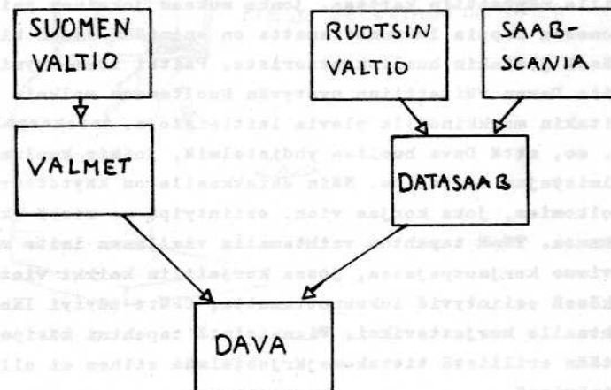
FIG 1. DATASAAB-VALMETIN OMISTUS-SUHTEET.
