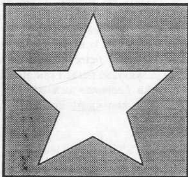
KUVA 1: Sirius-tähti
